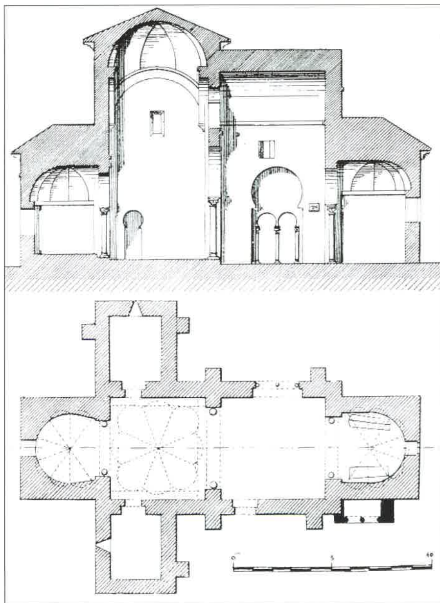
Fig. 2. Planta y sección de Santiago de Peñalba (según Luengo).
